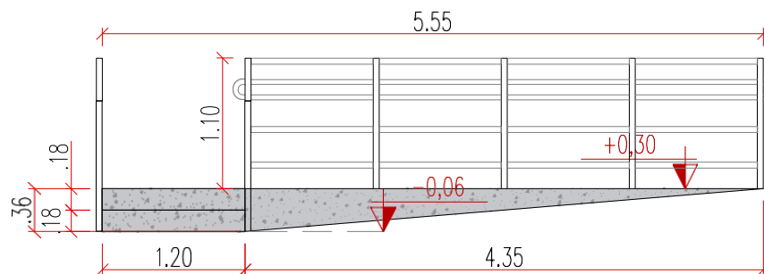
RAMPA DE ACESSO FÁRMACIA - UPA CENTRAL ELEVÇÃO FRONTAL ESCALA 1:50
