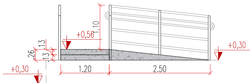
RAMPA DE ACESSO SALA DE TRIAGEM - AME CENTRAL ELEVÇÃO FRONTAL ESCALA 1:50
