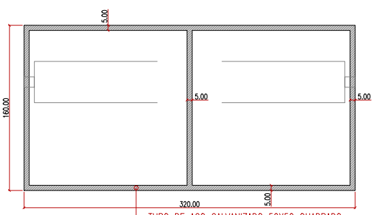
PONTO DE ÔNIBUS PLANTA NÍVEL +2,05 (BASE DO TELHADO)
