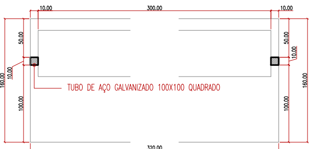
PONTO DE ÔNIBUS PLANTA NÍVEL +0,25
