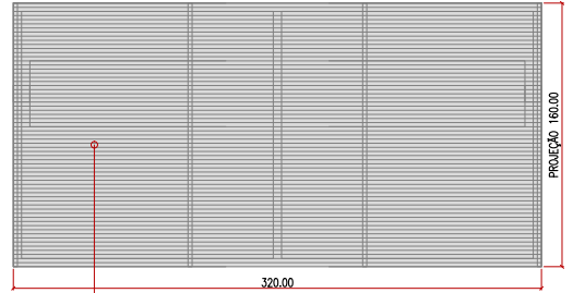
PONTO DE ÔNIBUS PLANTA DE COBERTURA
