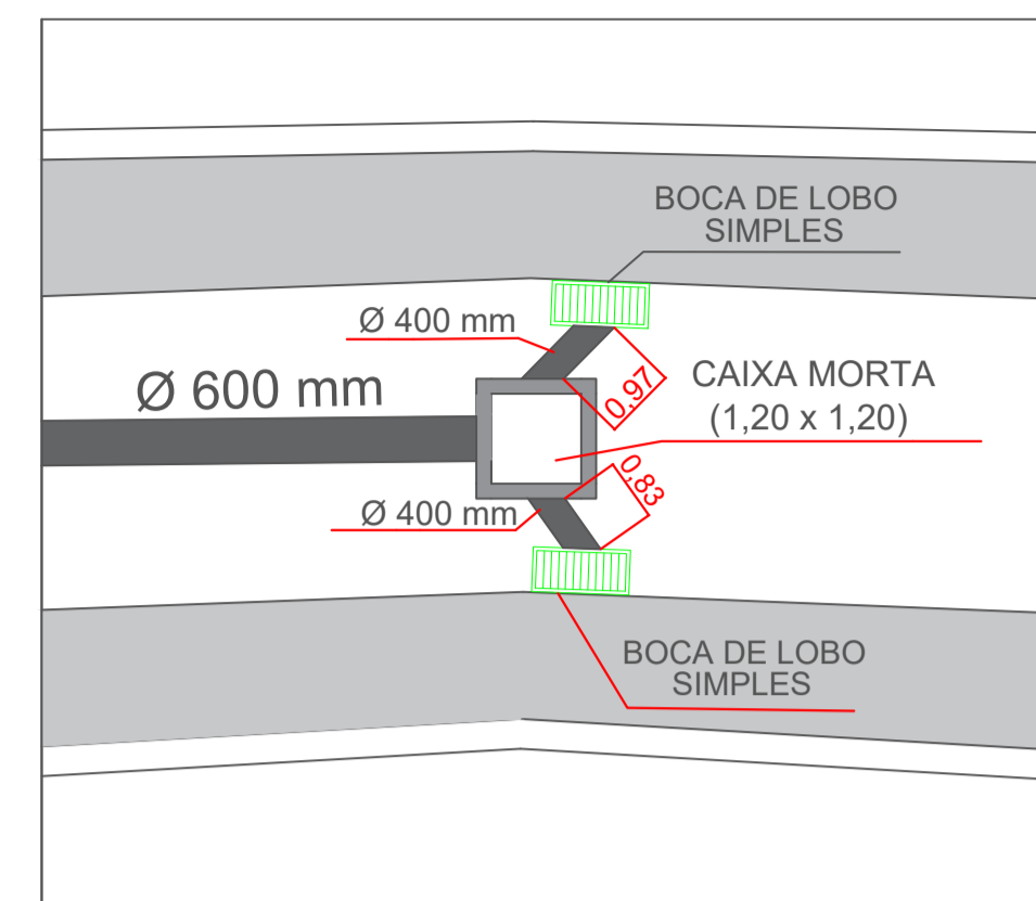
DETALHAMENTO DO SISTEMA DE DRENAGEM COM BOCA DE LOBO SIMPLES SEM ESCALA
