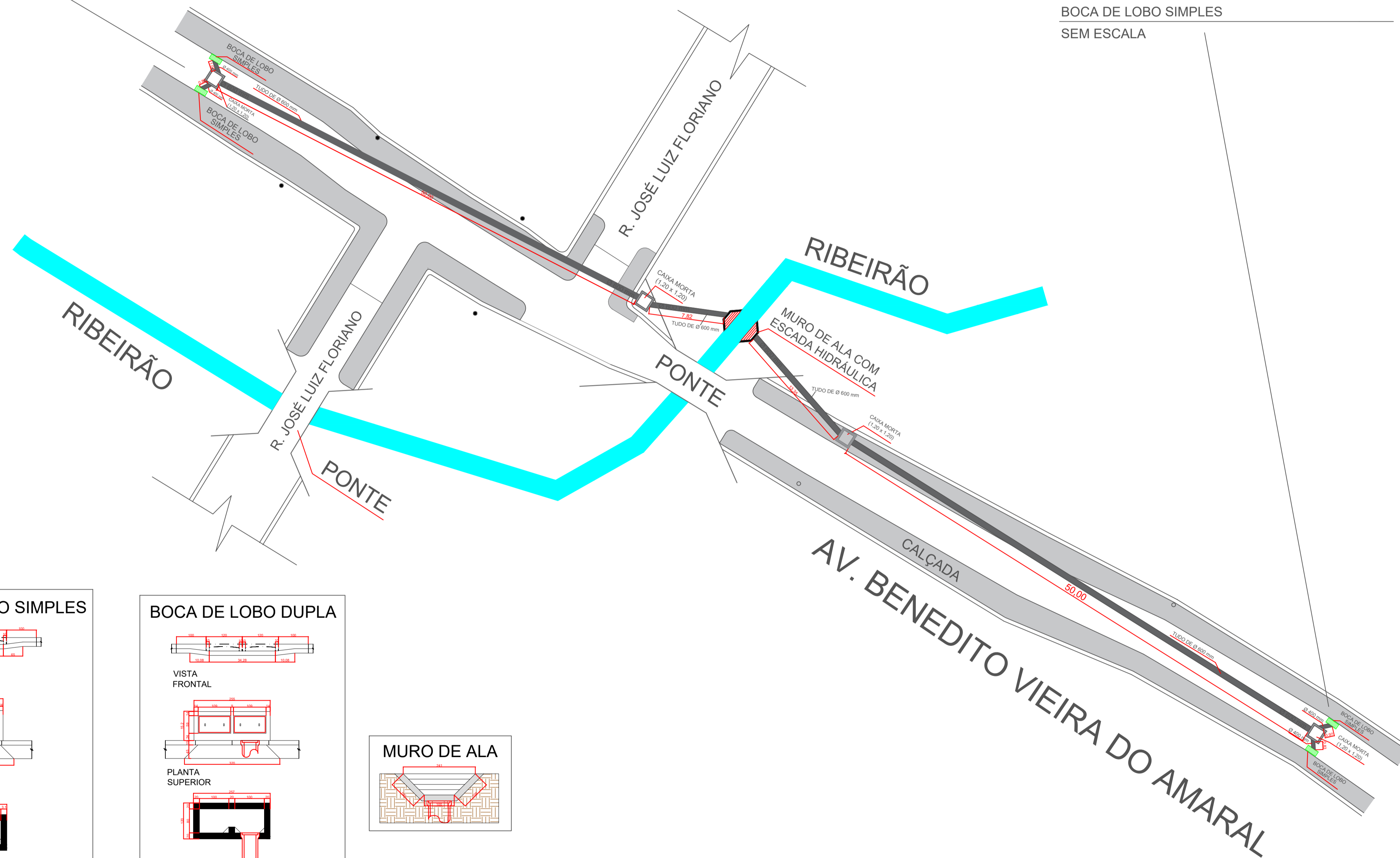
DETALHAMENTO DO SISTEMA DE DRENAGEM COM BOCA DE LOBO SIMPLES SEM ESCALA
