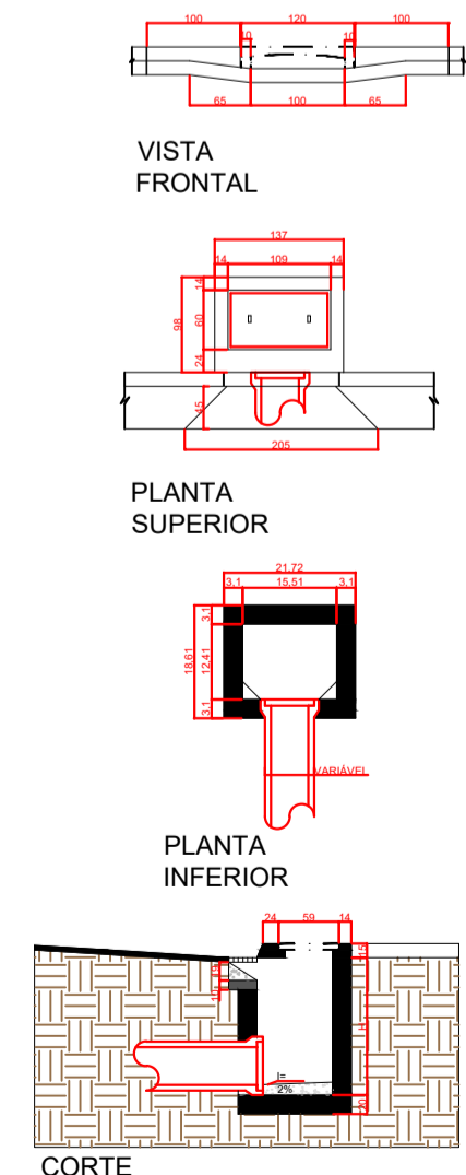
DETALHAMENTO BOCA DE LOBO E MURO DE ALA SEM ESCALA
